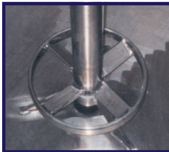
Elica chiusa a 4 pale
