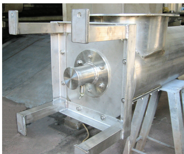
Coclea verticale, supporto di fondo a bicchiere
