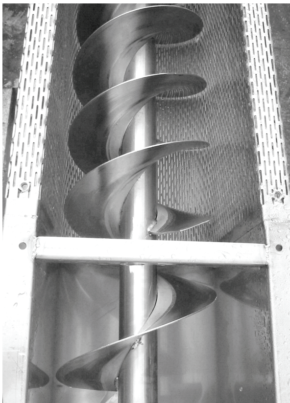
Elica a due principi nella zona di sgrondo
