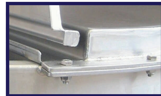
Particolare sportello igienico
